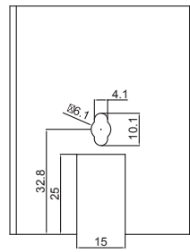
LAVORAZIONE MACHINING
