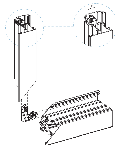
art. 0145 /.2/.3/.4/.5 Giunzioni angolari Corner joints
