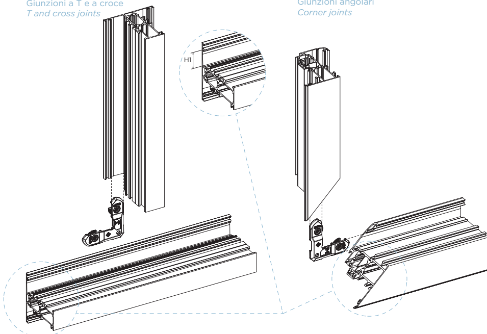
art. 0145.101 /.102 Giunzioni angolari Corner joints
