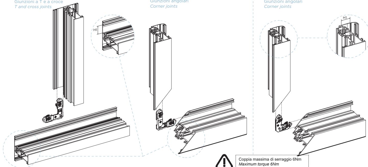
art. 0145.101 /.102 Giunzioni angolari Corner joints
