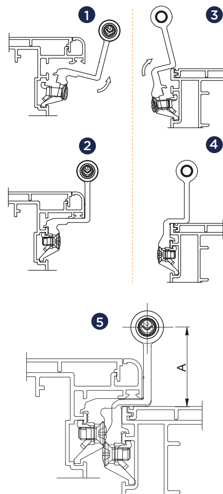
MONTAGGIO VERSIONE TOP RAPID ASSEMBLING TOP RAPID VERSION
