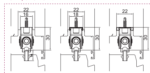
SPESSORE CARRELLO | THICKNESS ROLLER
