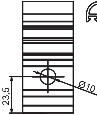
Lavorazione Anta R40 Machining Sash R40
