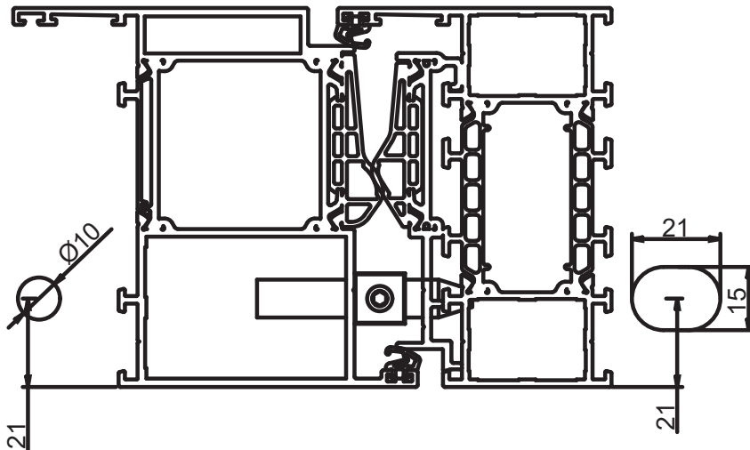
Lavorazione Telaio PORTA Machining Sash DOOR
