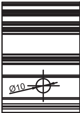
Lavorazione Anta CE Machining Sash CE
